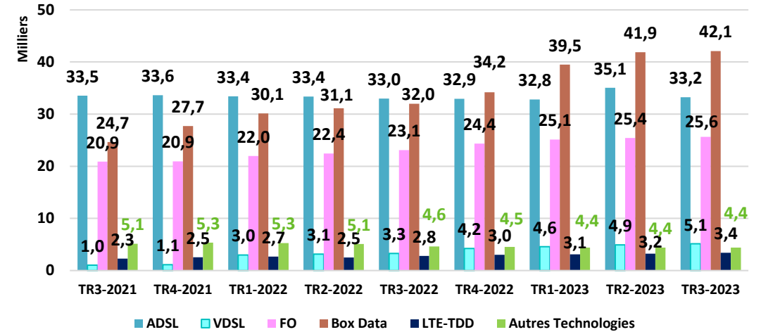
Abonnements PRO data fixe par technologie
